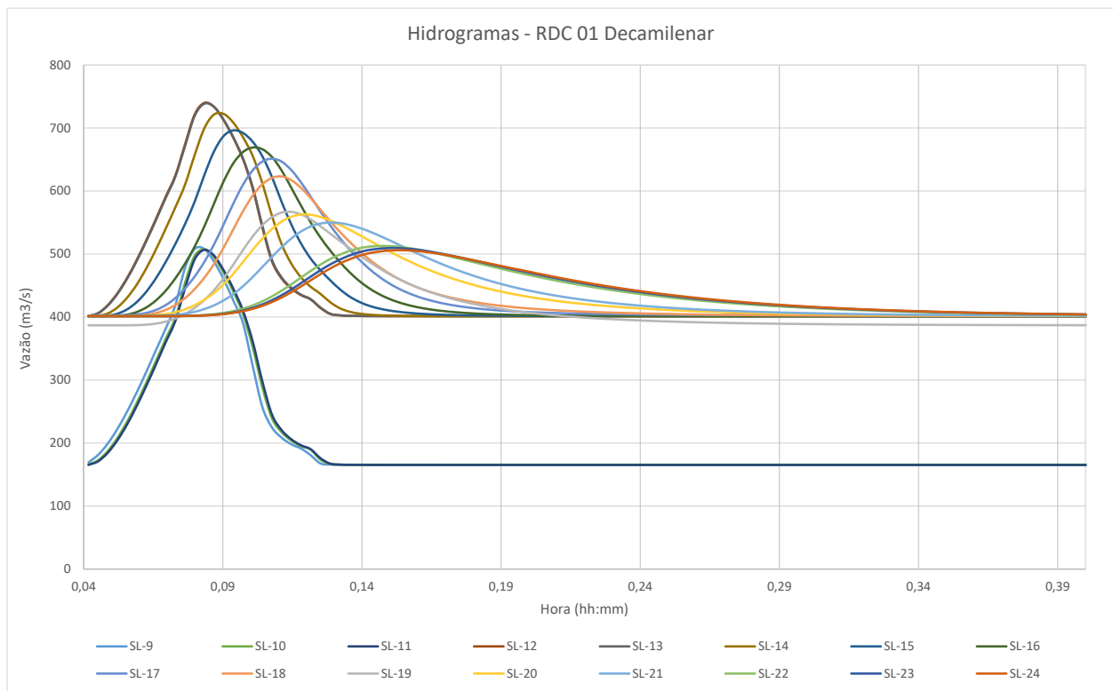
Figura 22 - Propagação de hidrogramas nas seções de controle Rio Jucuruçu do Sul RDC 1 (Decamilenar).
