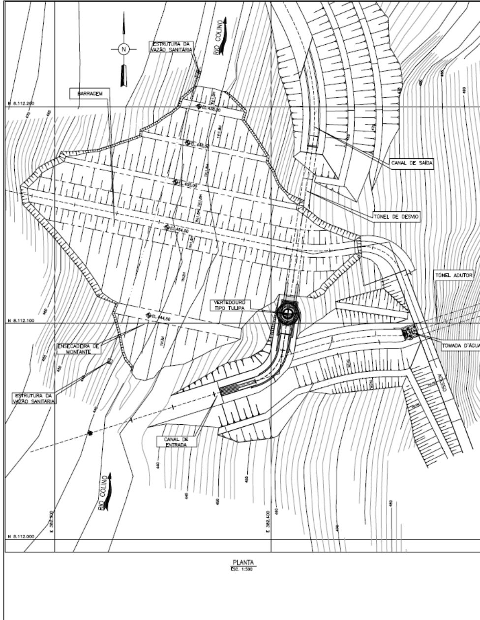
Figura 10 – Arranjo Geral de Montante
