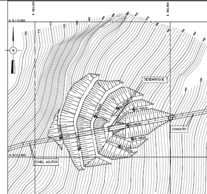
PLANTA Esc. 1:500
