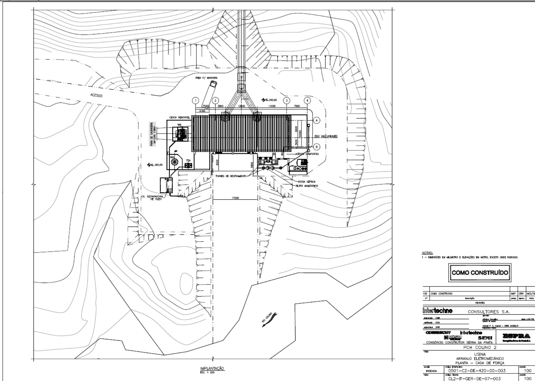
Figura 16 – Planta Casa de Força
