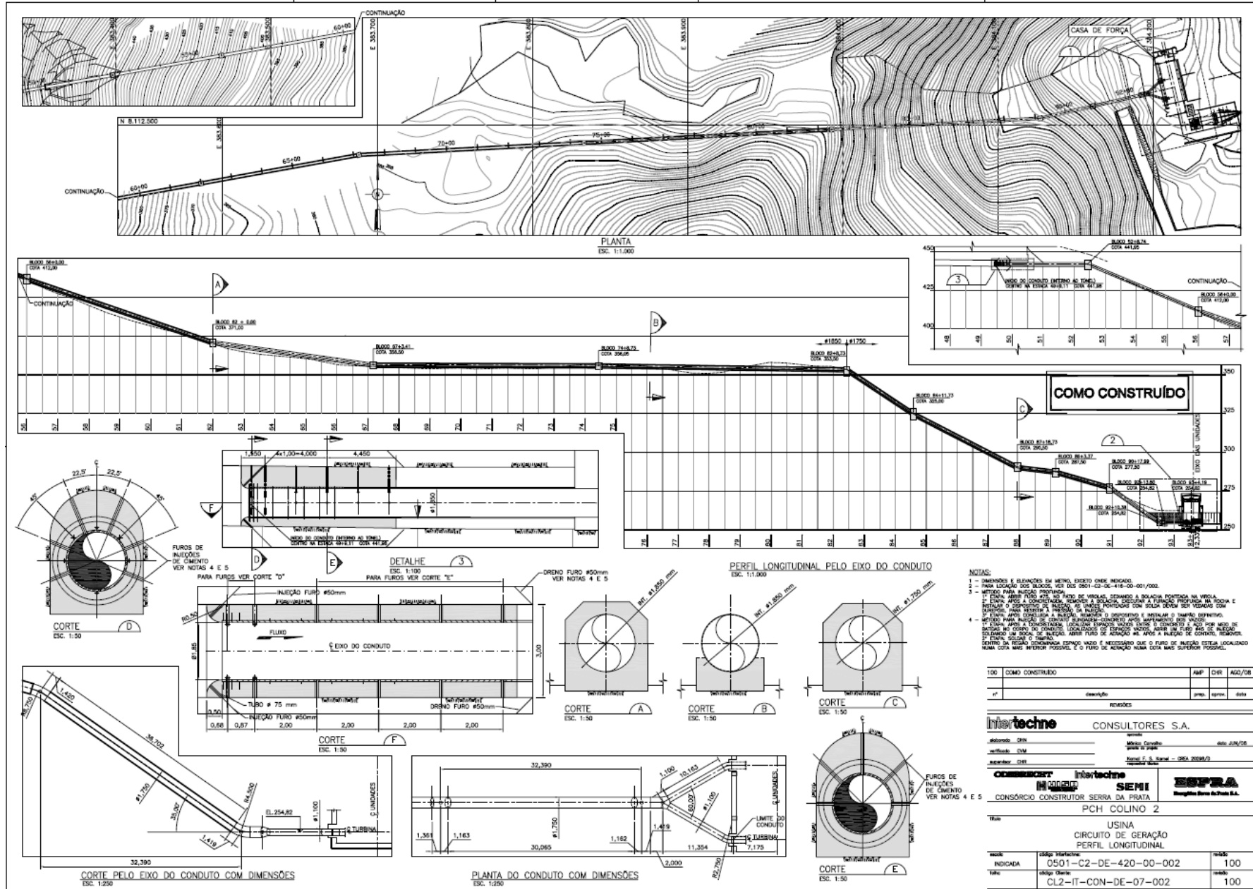
Figura 15 – Circuito de Geração - Planta e Seção
